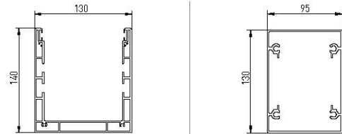
Viga frontal
